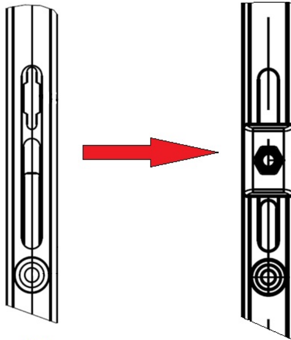
Rys. 1 Sztancowanie na zasuwnicy skrzydła biernego
