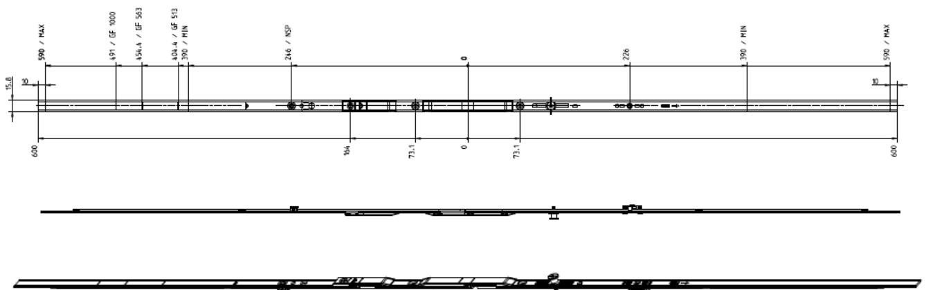
Rysunek zasuwicy 795349 - NX Zas.adapt.M EasyMix 0810-2400 1V+PZ
