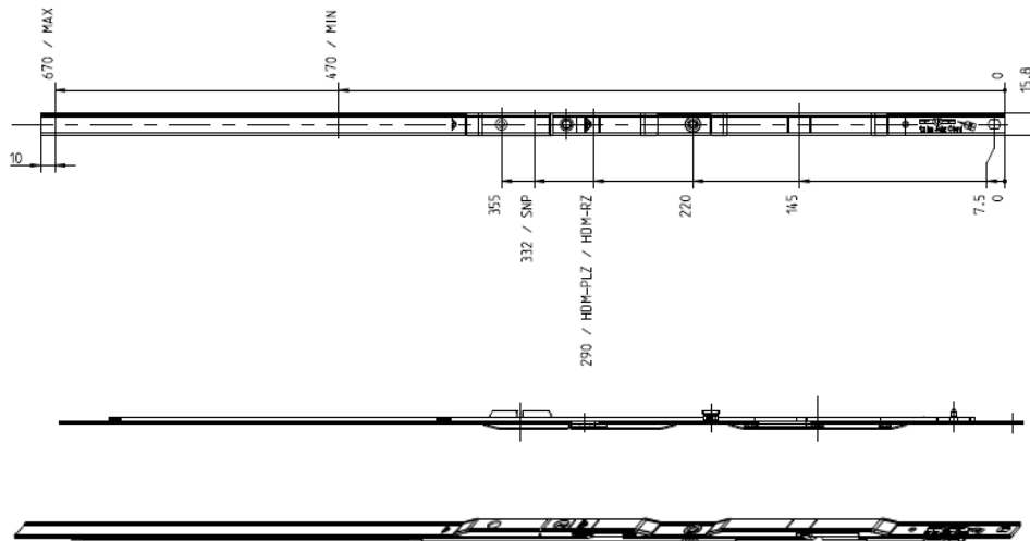
Rysunek zasuwicy 799011 - NX Zas.adapt.M EasyMix 0690-2400+PZ
