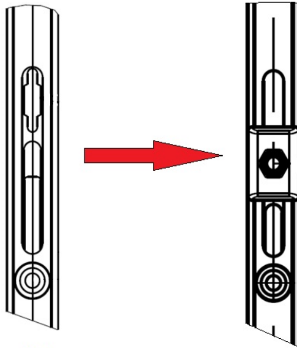
Rys. 1 Sztancowanie na zasuwnicy skrzydła biernego
